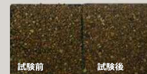
約20年相当アイスーパーUVテスター試験結果
